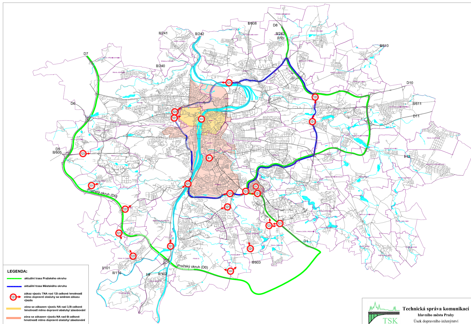
Obr. 1: Omezení jízdy NA nad 12 t celkové hmotnosti na vybrané komunikační síti na území hl. m. Prahy
